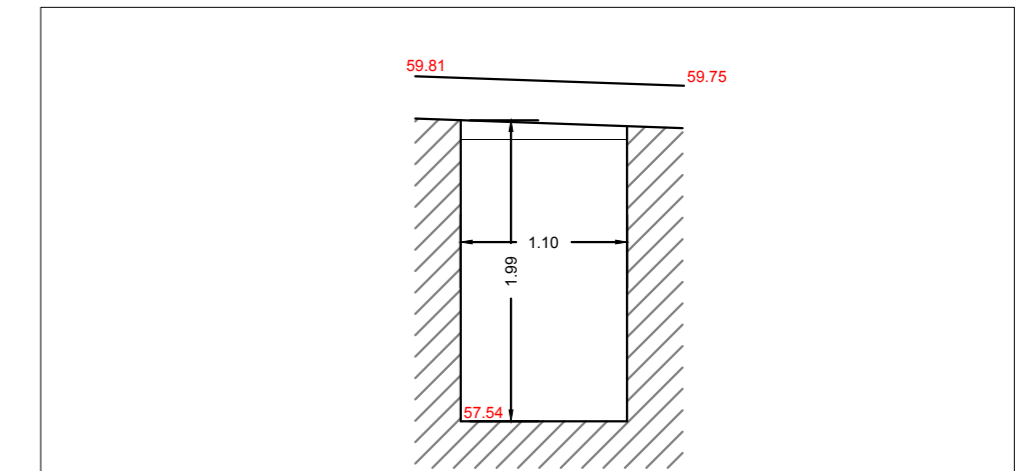
Ouvrage M3 AMONT
