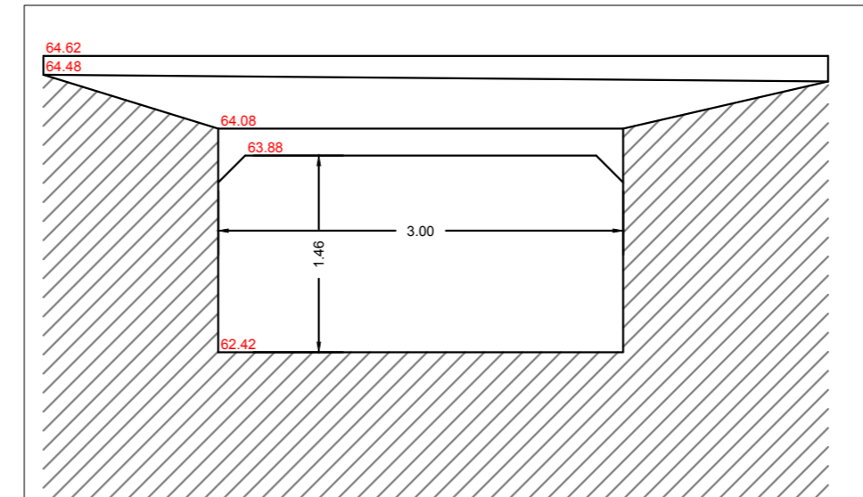
Ouvrage M2 AVA
