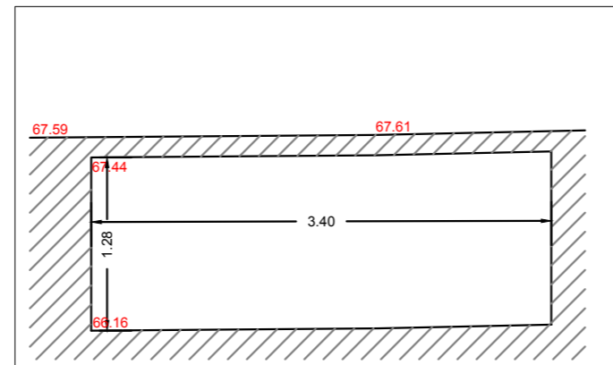
Ouvrage M1 AMONT
