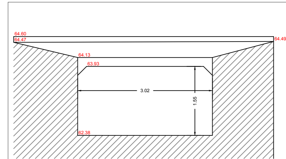
Ouvrage M2 AMONT
